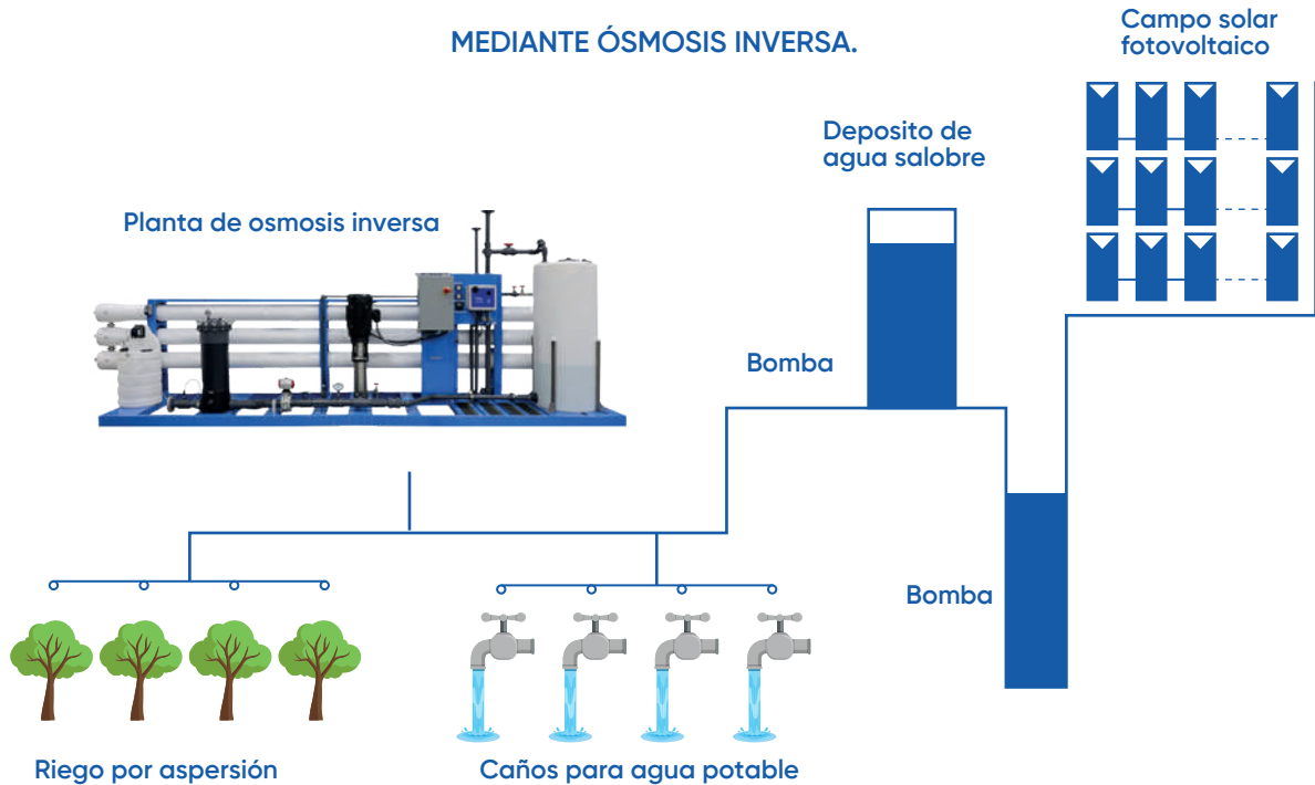
Proyecto bombeo solar realizado en Gambia (África)
